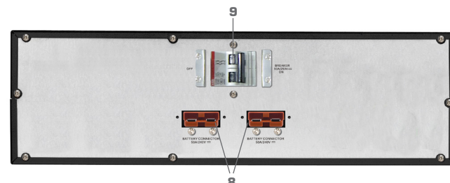
Module d'autonomie E7 One 8k/10k RT (3U)
