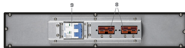
Module d'autonomie E7 One 5k/6k RT (2U)
