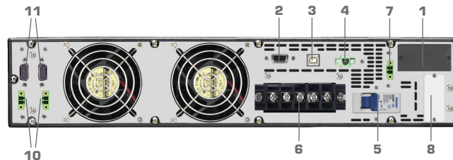
E7 One 5k, 6k & 10k RT
